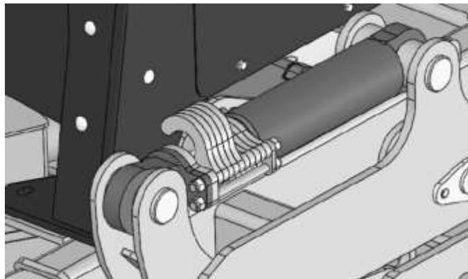
Rys. : 11 Podkładki na siłowniku
