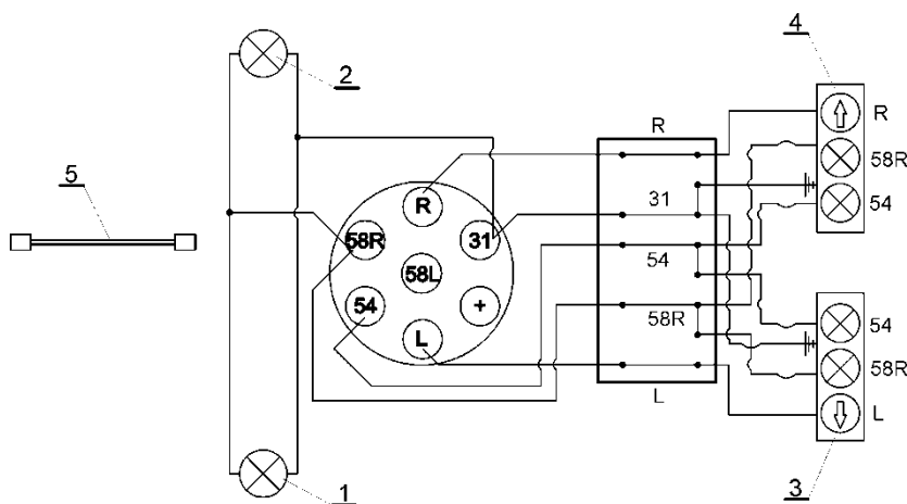
Rys.21 Schemat instalacji oświetleniowej
