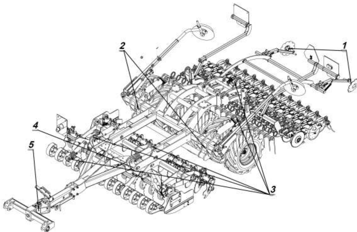
Rys.20 Schemat smarowania.
